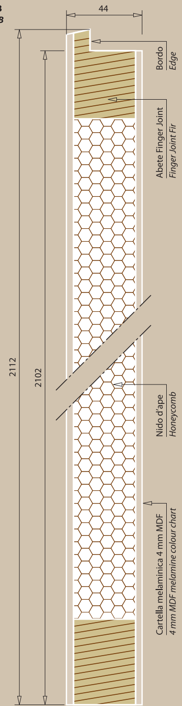
Sez. B - B Sect. B - B
